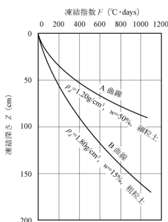
図 5-14 細粒土と粗粒土における凍結指数と凍結深さの関係 （寒冷地地盤工学 5-15) から引用）
