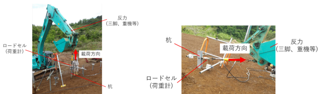
(a) 引抜き載荷試験の状況
