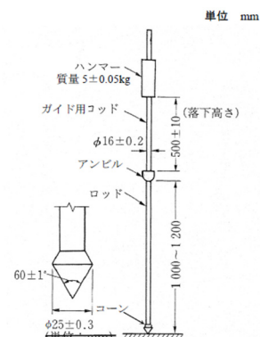
図 5-5 簡易動的コーン貫入試験機
