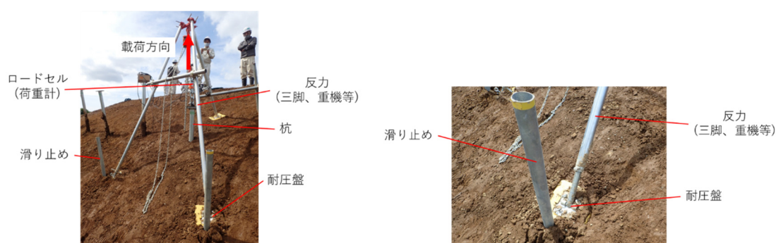
(a) 引抜き載荷試験の状況
