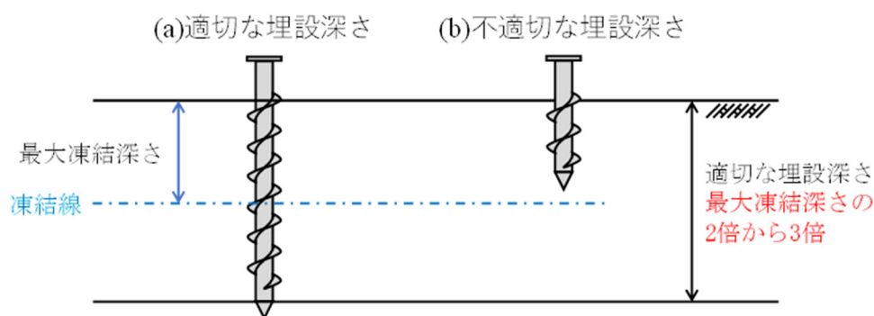
図 11-7 杭基礎の適切な埋設方法
