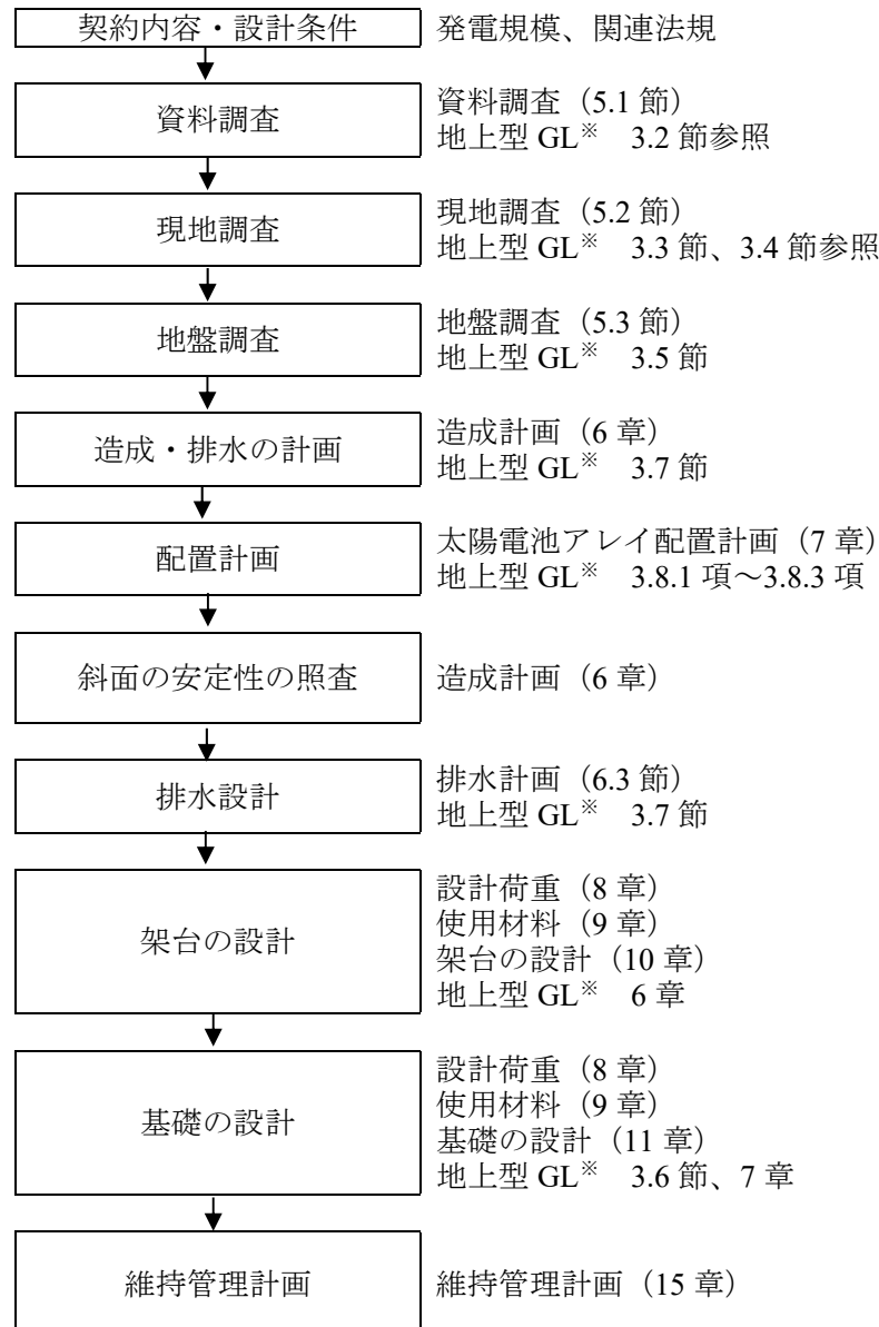
図 3-1 構造設計フロー
