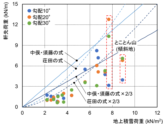
図 8-6 実証実験で得られた地上積雪荷重と軒先荷重との関係
