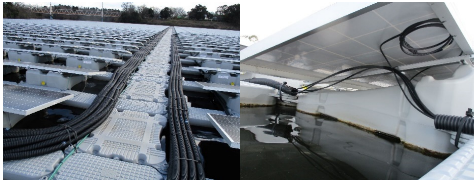
写真 12-2 配管に納めた配線の例
