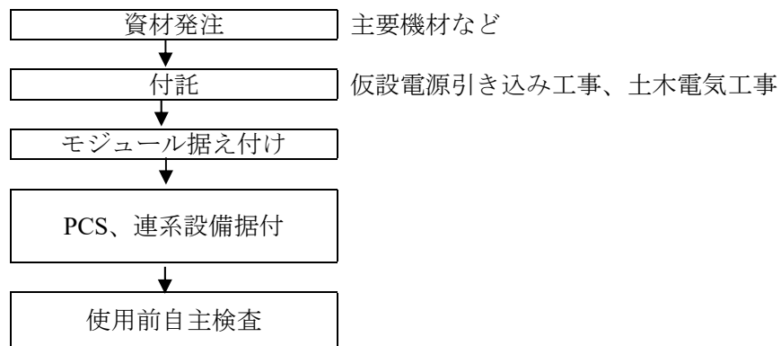
図 4-2 施工フロー（電気） 4-1)
