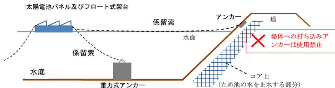
図 10-5 堤体への打込式アンカーの使用を禁止としている事例 10-2)
