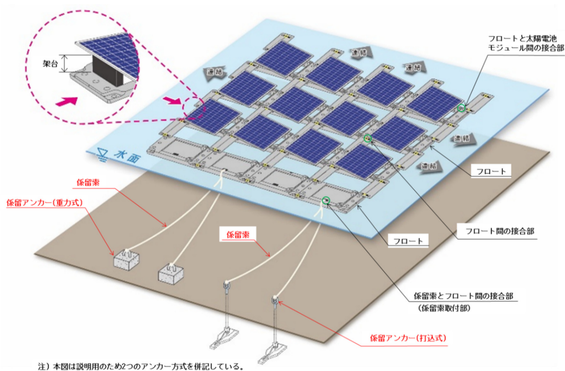
図 10-1 係留設計の対象部材
