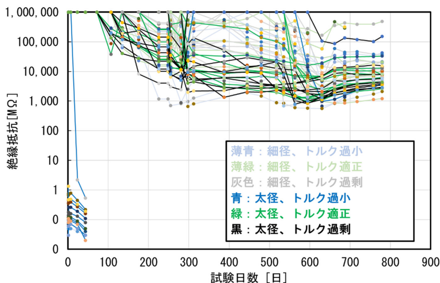
図 12-1 コネクタのトルクと線径別の浸水試験結果
