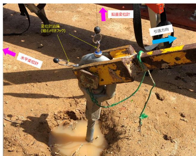
図 4-2 変位計の計測点（スイベルアイナット、試験前）
