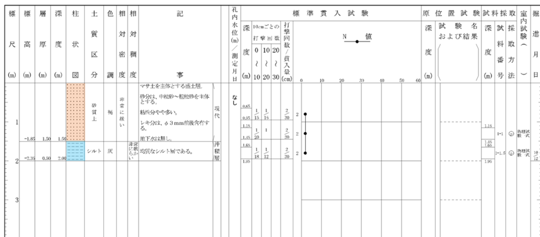
図 3-7 柱状図 Bor. No. 1
