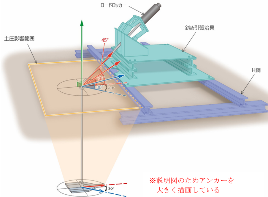
図 4-1 斜め引張治具の配置
