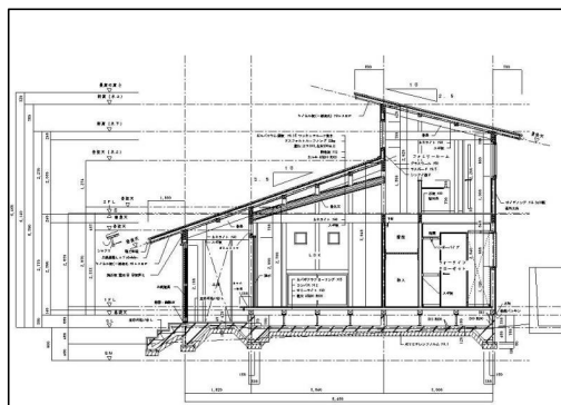
矩計図 (かなばかりず)
