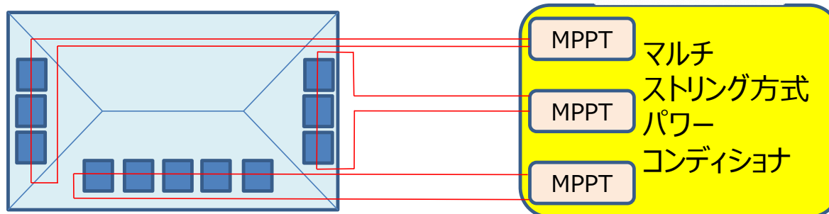
マルチストリング式パワーコンディショナ
