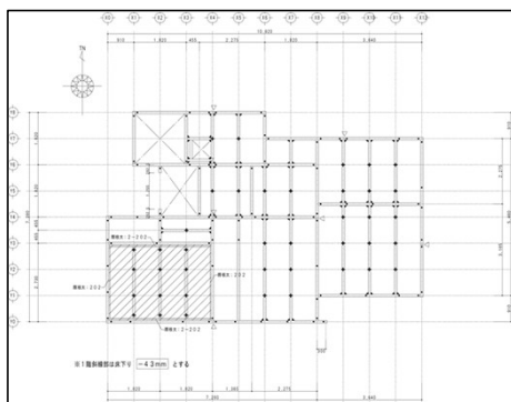
屋根伏図
