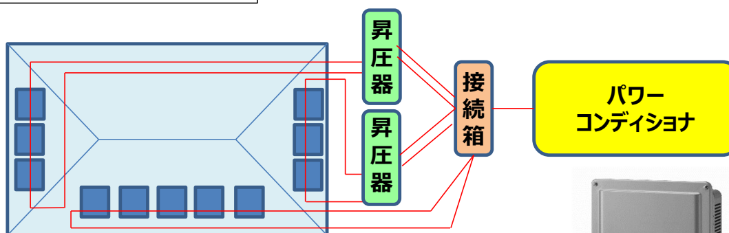
一般的なパワーコンディショナ
