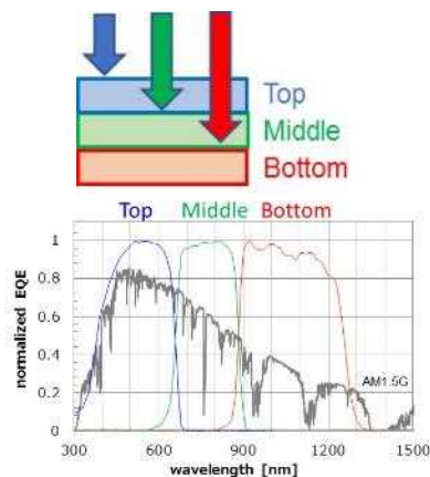
各要素セルの量子効率(EQE)
